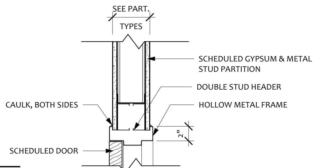
DOOR HEAD DETAIL @ STUD WALL
