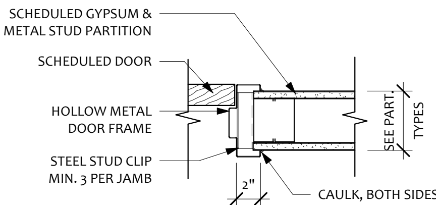
DOOR JAMB DETAIL @ STUD WALL
