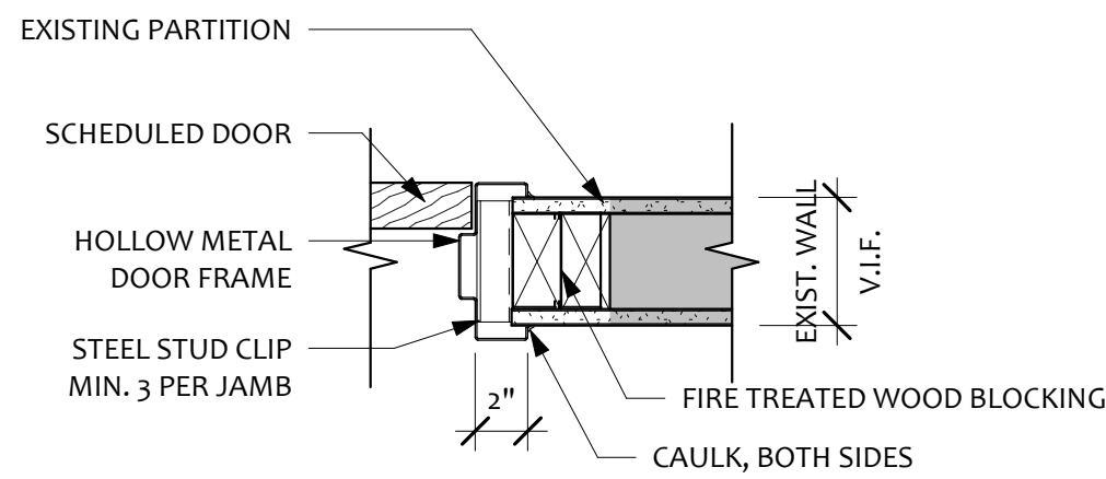
DOOR JAMB DETAIL @ STUD WALL
